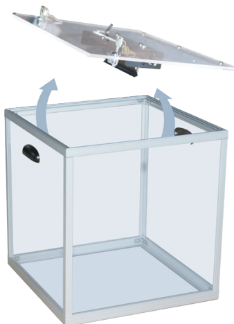
Urne jusqu'à 1200 bulletins Format : 400 x 400 x H 420 mm (Réf. SPL527110)
